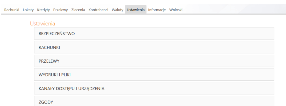
Rys. 43 Okno „Ustawienia”
